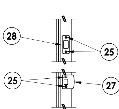
LATCH & DEADBOLT DETAIL Schlage / Kwikset
